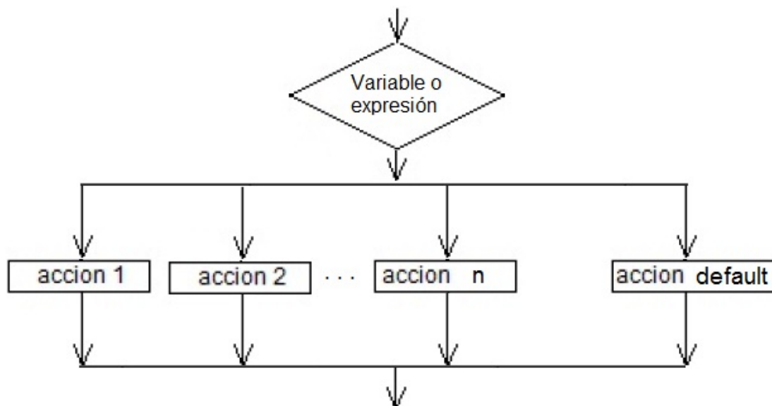
Figura 6. Estructura switch case (según caso)
