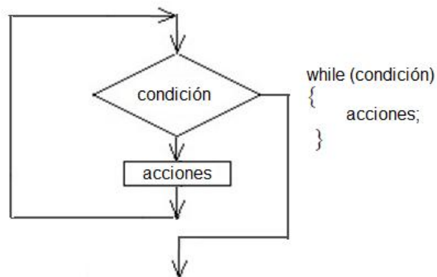
Figura 8. Estructura while
